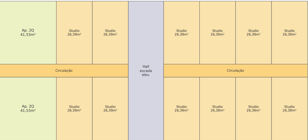
Pavimento Tipo 2 2Q + 12 studios (7x)
